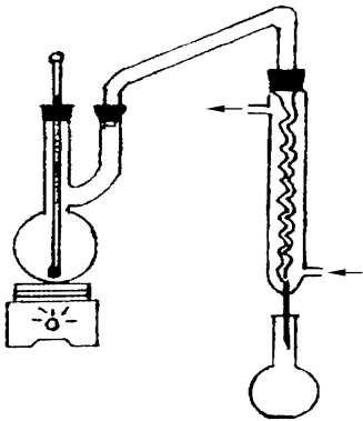
图 3 氟化物蒸馏装置
