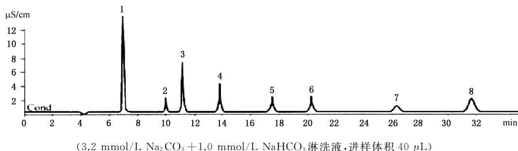
图 7 用 Metrosep A Supp 5-250 分析柱分离的混合标准溶液的色谱图
