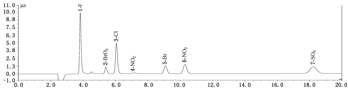
图 7 用 IonPac AS9-HC 分析柱分离的混合标准溶液的色谱图 (7.2 mmol/L \text{Na}_2\text{CO}_3 + 2.0 mmol/L NaOH 淋洗液,进样体积 100 \mu\text{L} )
