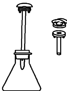
图 3 砷化氢发生吸收装置图
